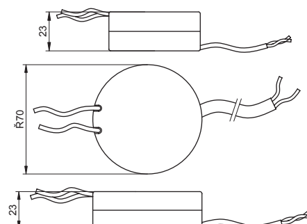
TRN-105R
