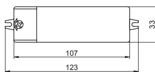
TRN-70
